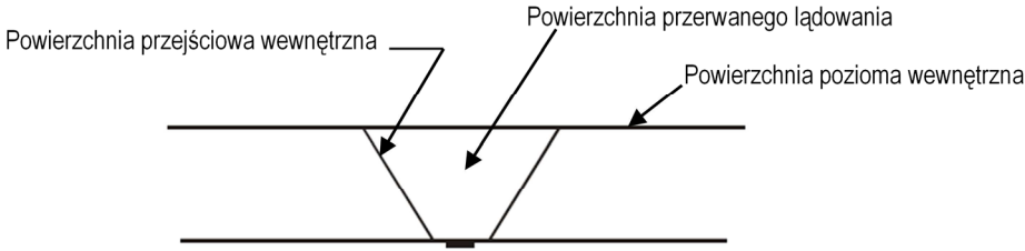
Przekrój B-B
