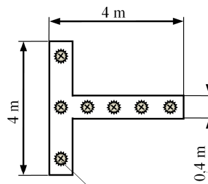
Światła wskaźnika kierunku lądowania: dookólne, koloru białego, minimum 7 sztuk (rozmeszczone równomiernie)
