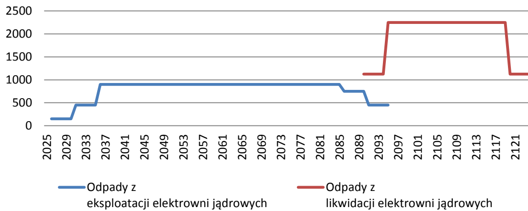
Rys.3.3. Prognoza ilości odpadów promieniotwórczych stałych nisko- i średnioaktywnych obejmująca lata 2025-2124, pochodzących z energetyki jądrowej [m 3 ]
