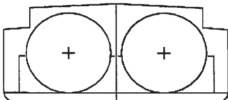
Typ N Stan zbiorników ładunkowych 2, 3 i 4 Typ zbiornika ładunkowego I (także jako gładkopokładowe)
