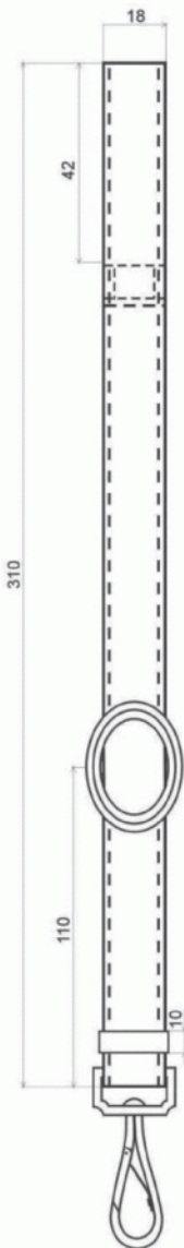
WYMIARY widok z przodu
