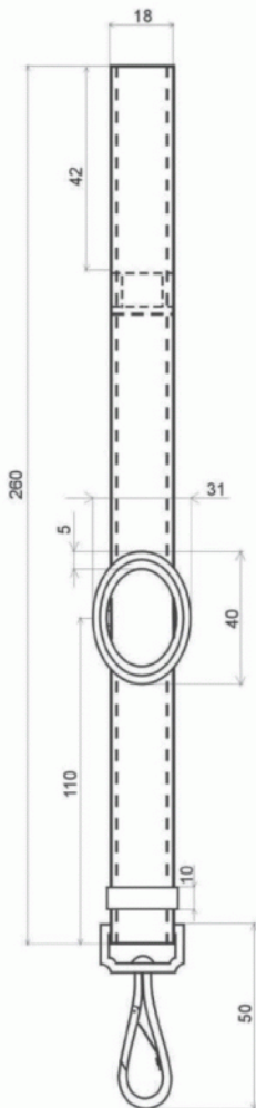
WYMIARY widok z przodu
