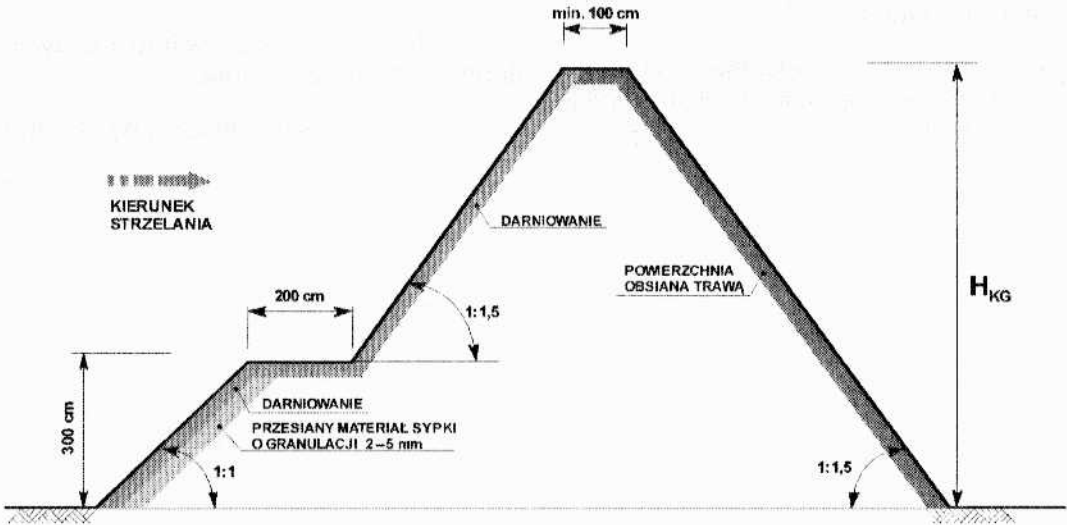
Rys. nr 1 Schemat ziemnego kulochwytu głównego
