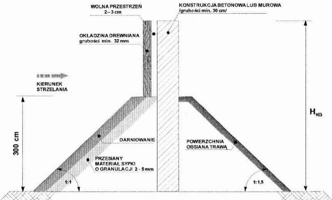
Rys. nr 2 Schemat ziemnego kulochwytu głównego o konstrukcji betonowej lub muruwej
