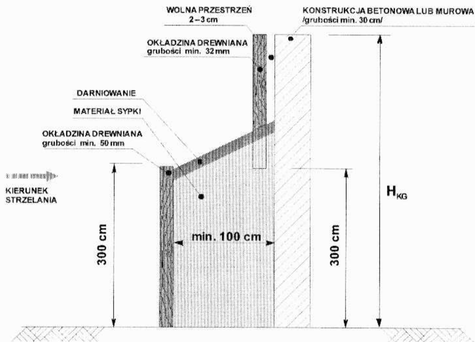
Rys. nr 3 Schemat kulochwyty głównego o konstrukcji betonowej lub murowej osłoniętej materiałem sypkim i okładziną drewnianą
