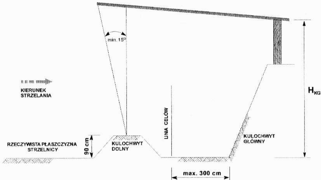
Rys. nr 5 Schemat zabudowy kulochwyty główny
