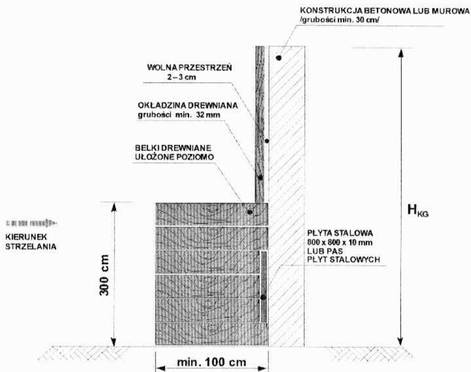
Rys. nr 4 Schemat kulochwyty głównego o konstrukcji betonowej lub murowej osłoniętej drewnem
