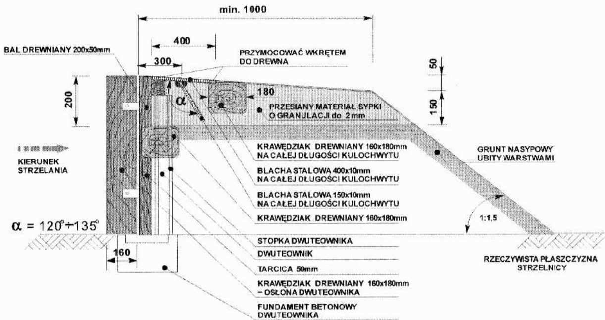
Rys. nr 6 Schemat kulochwyty dolnej pod przestoną pionową nr 1 (wymiar w mm)
