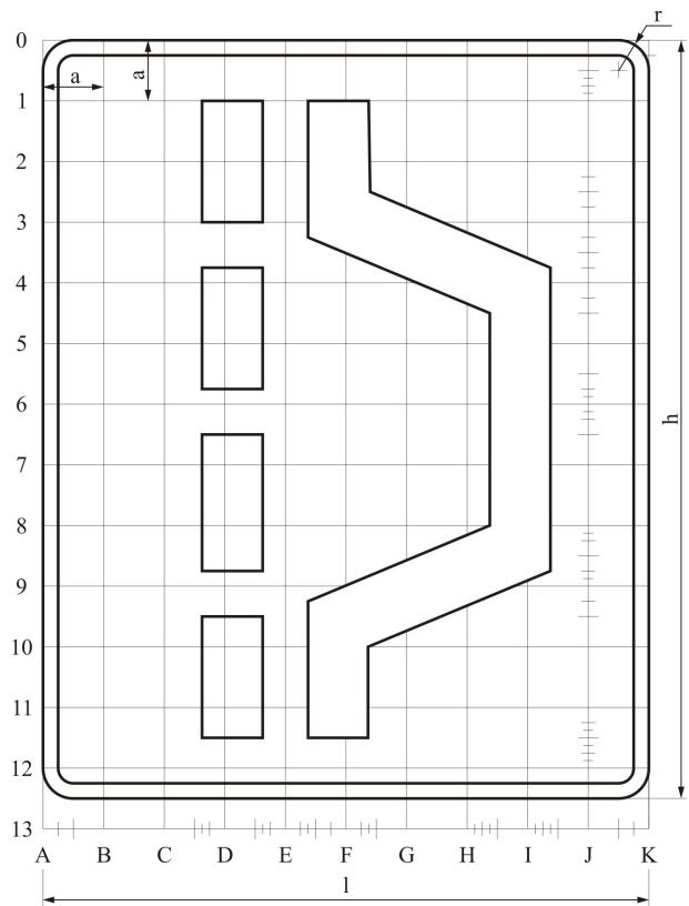
Wymiary h, l, r - zgodnie z tabelą 5.1
