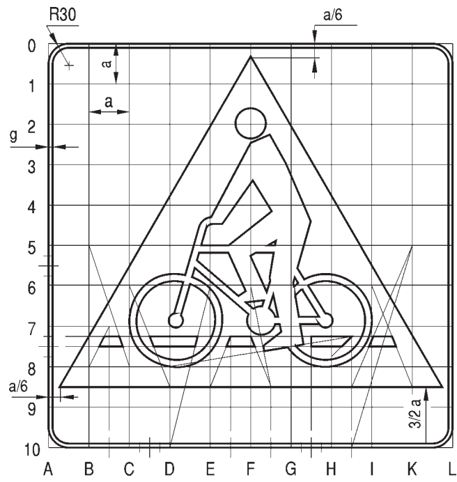
Szablon roweru według konstrukcji na rys. 9.3.7.
