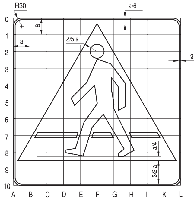
Sylwetka pieszego według konstrukcji na rys. 9.1.18.
