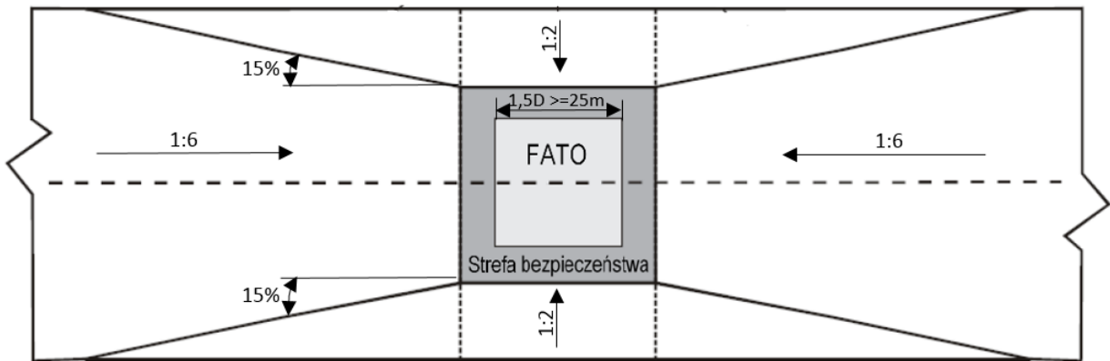
Rzut poziomy
